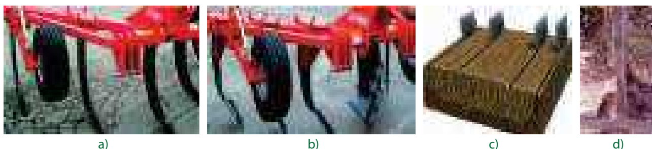
Fig. 5.9. Formele trupițelor: a) dreaptă; b) încovoiată; c) schema afânării cu paraplow; d) trupița centrală uzată
