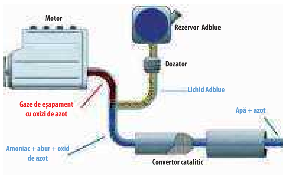
Fig. 5.7. Sistemul cu lichid Adblue de reducere catalitică selectivă a substanțelor nocive
