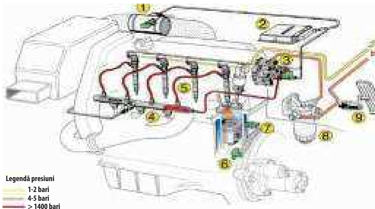
Fig. 5.5. Sistem de injecție cu rampă comună (Virubov D., 2018): 1 – debitmetru de aer; 2 – procesor injecție; 3 – pompă de înaltă presiune; 4 – rampă comună; 5 – injectoare; 6 – senzor turație motor; 7 – senzor temperatură motor; 8 – filtru motorină; 9 – senzor poziție pedală de accelerație
