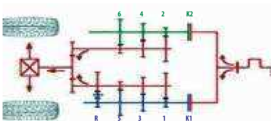
Fig. 5.6. Fluxul de putere în transmisia Powershift (Wimmer, 2016)
