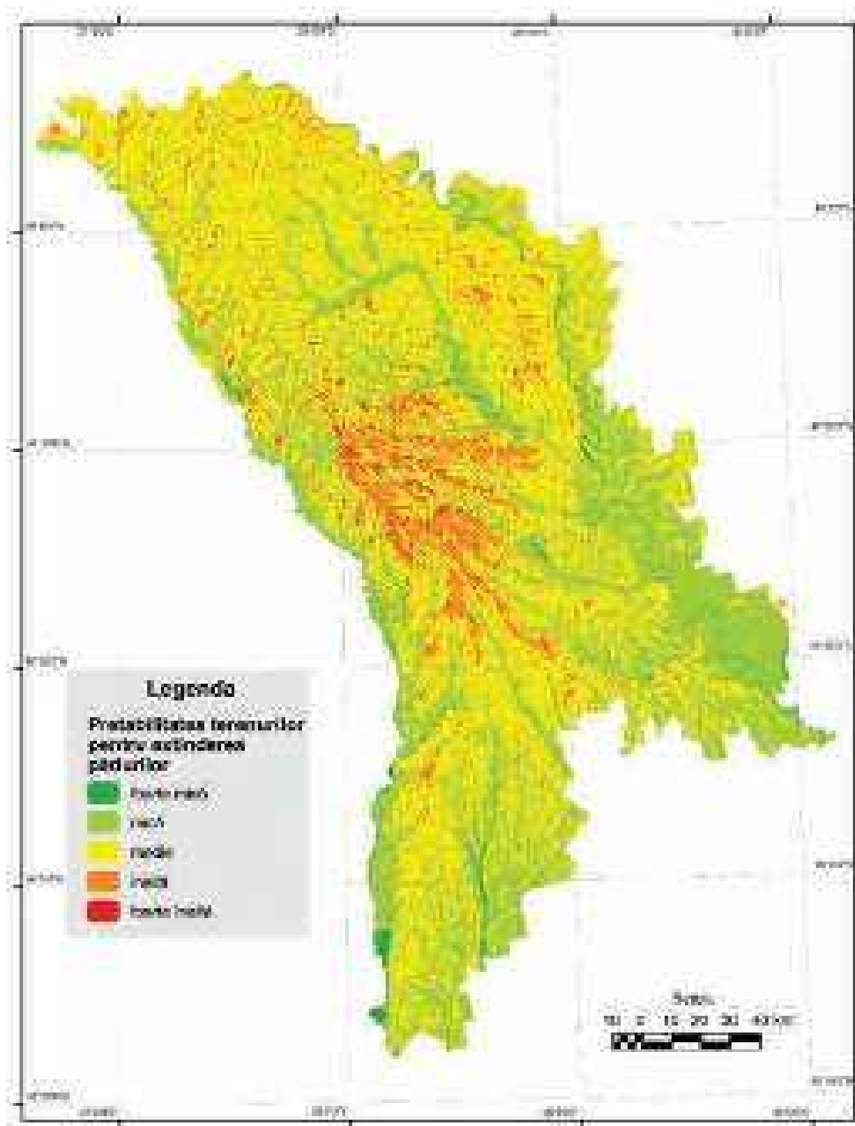
Fig. 7.3. Preabilitatea teritoriului Republicii Moldova la împădurire
